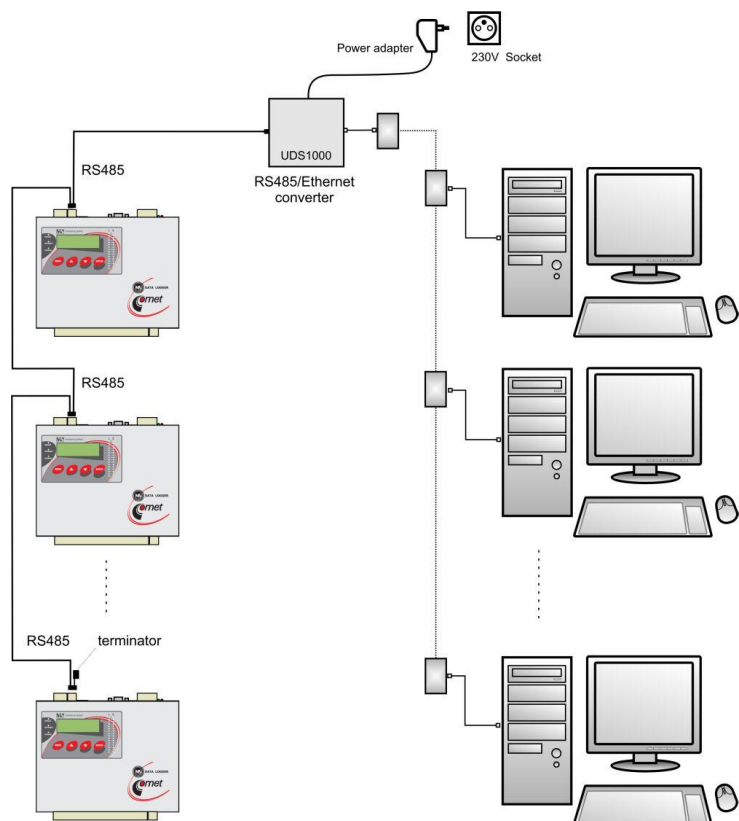
Schéma propojovacího kabelu mezi ústřednou převodníkem RS485/Ethernet Lantronix UDS10/100/1000:
