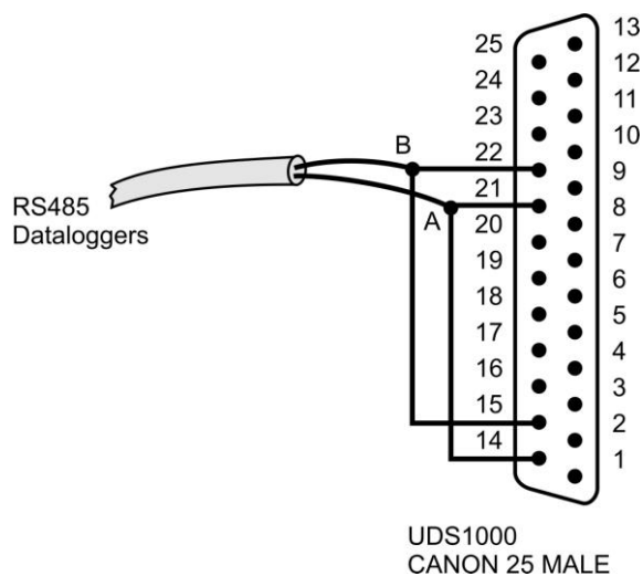
Schéma propojovacího kabelu mezi ústřednou převodníkem RS485/Ethernet Lantronix UDS10/100/1000:
